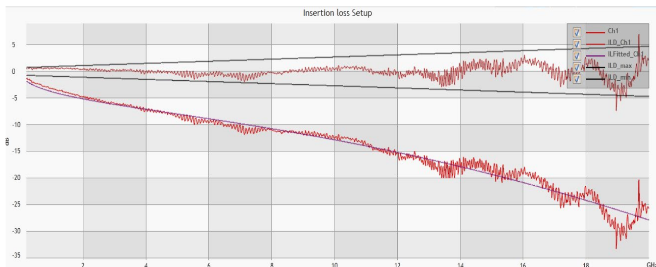
Figure 17: ILD & IL Fitted
